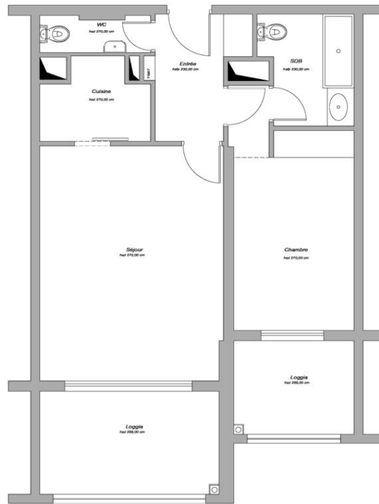
Lucio & Vito Di Rosa Apt.94b Rosa Maris, Monaco Pianta generale / Stato Attuale 1:25 Apr 2024 / Disegno No. 01
