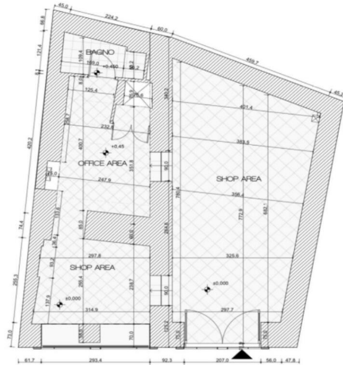
PLANIMETRIA STATO ATTUALE 1:50
