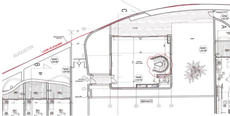
ELLA ETAGE 3 | Bâtiment C - Rez de chaussée - éch: 1/100e
