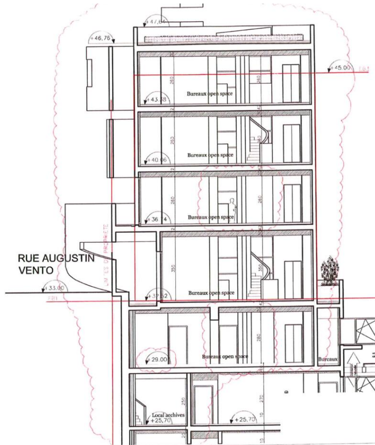
Bâtiment C - Coupe C-C' - éch: 1/100e
