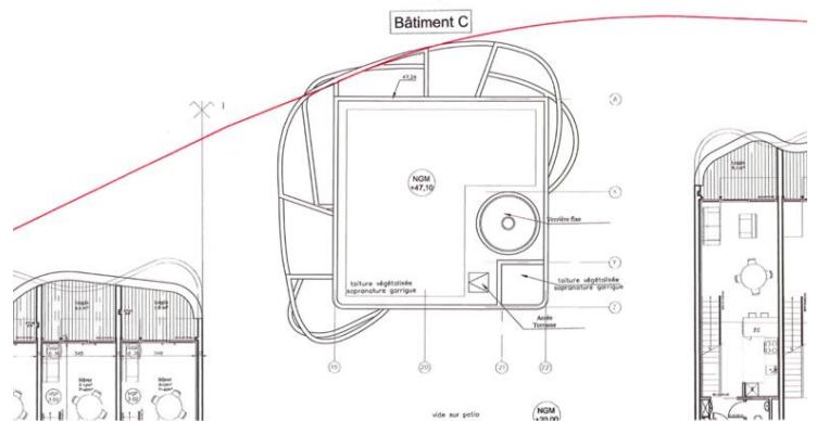
ELLA ETAGE 7 | Bâtiment C -Toiture-éch: 1/100e
