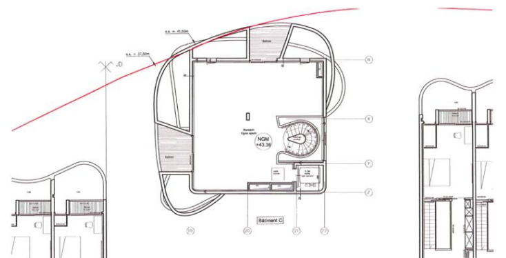
ELLA ETAGE 6 | Bâtiment C-Etage 3 -éch: 1/100e
