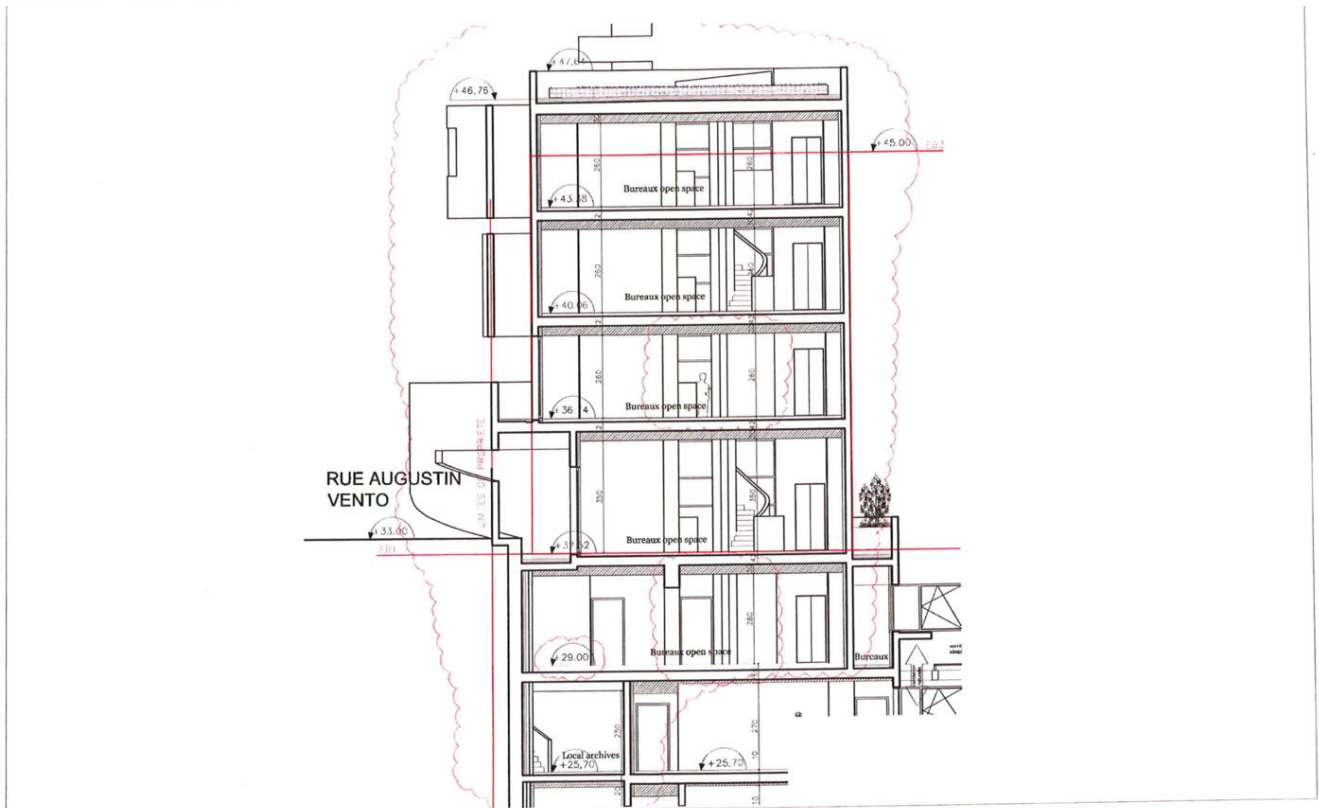
Bâtiment C - Coupe C-C' - éch: 1/100e
