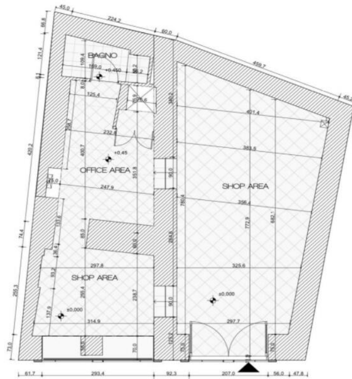
PLANIMETRIA STATO ATTUALE 1:50
