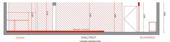
Coupe - Etat projeté
