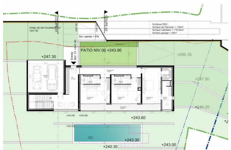
GUILHEM & CARBONE Architecture VILLA B Parcelle AK 4.6 Chemin de Grima - 06240 BEAUSOULEL PLAN NIVEAU 01 / ETAGE VILLA - ACCES APB 06 Echelle: 1:100 Date: 20/03/2021
