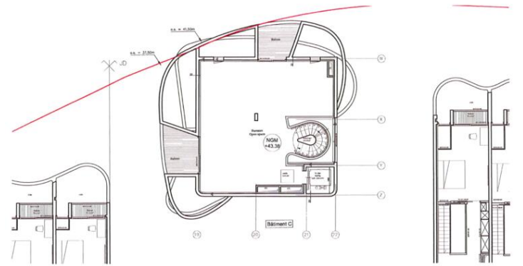
ELLA ETAGE 6 | Bâtiment C-Etage 3 -éch: 1/100e | mai 2014
