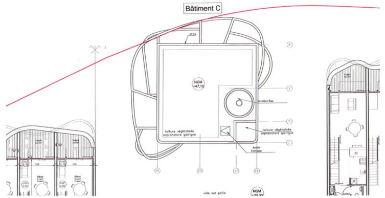
ELLA ETAGE 7 | Bâtiment C -Toiture-éch: 1/100e | mai 2014
